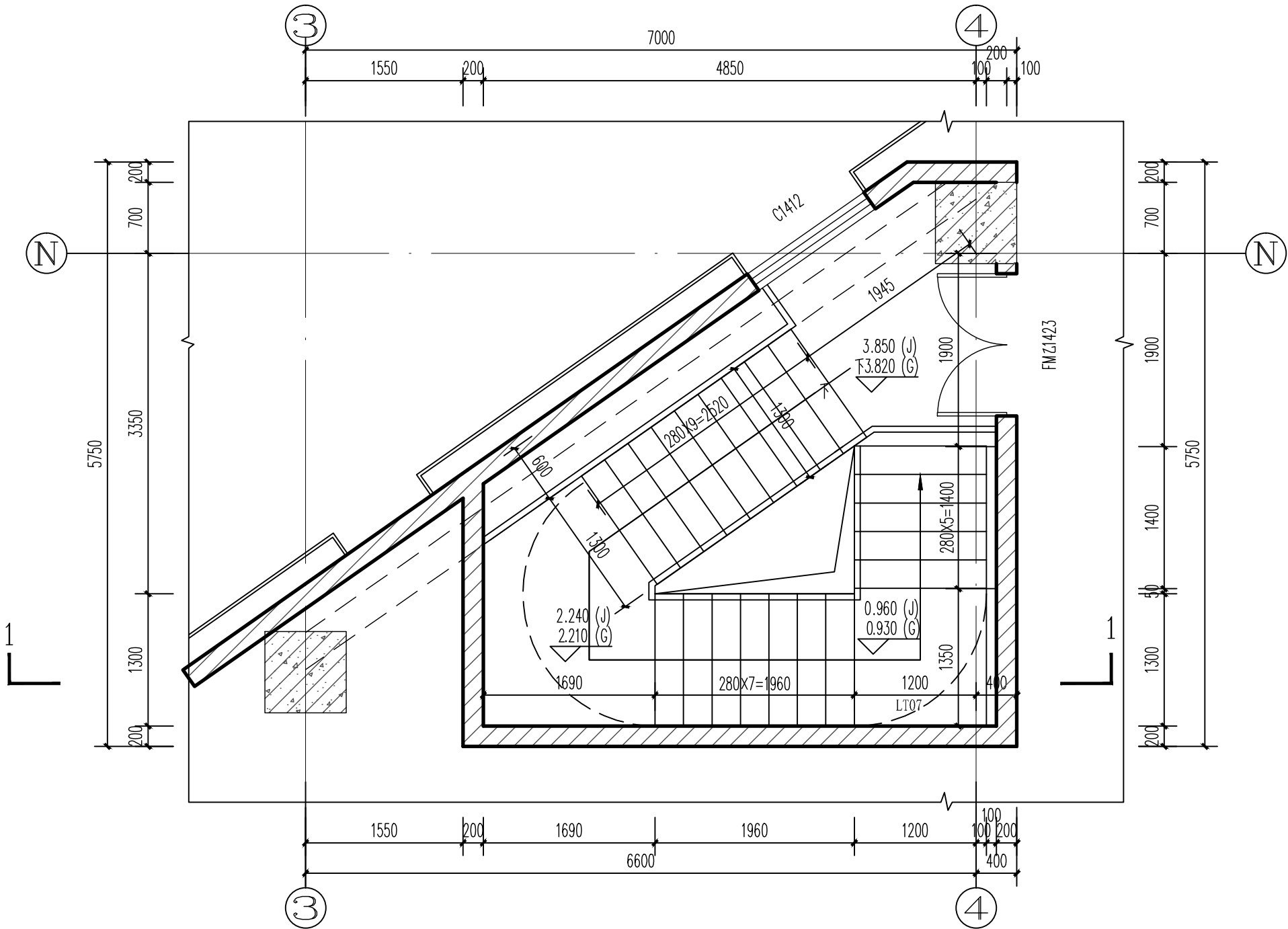
LT08 首层夹层平面
